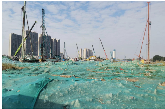
● 顺德乐从小布碧桂园基础工程
